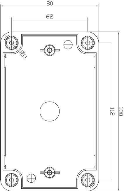
图3 急停套装盒体尺寸
