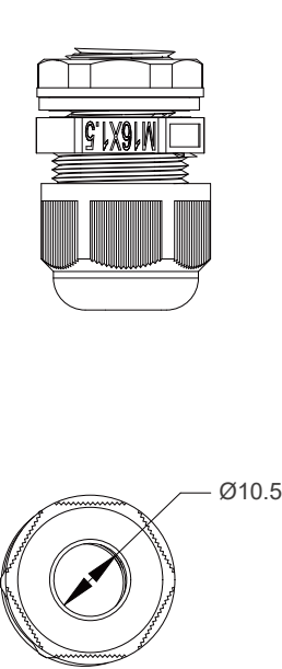
图4 防水接头尺寸
