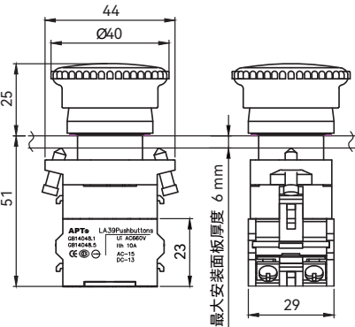
图2 按钮的外形尺寸
