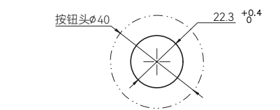
图1 按钮的安装孔尺寸
